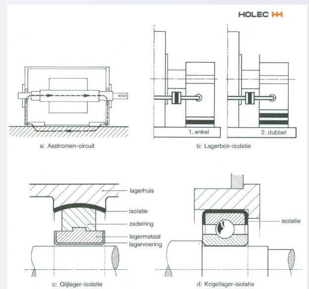
Afbeelding 1. Asstroomcircuit en lagerisolatie. (Bron: Holec)
